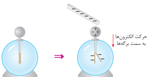
الکتروسکوپ خنثی
